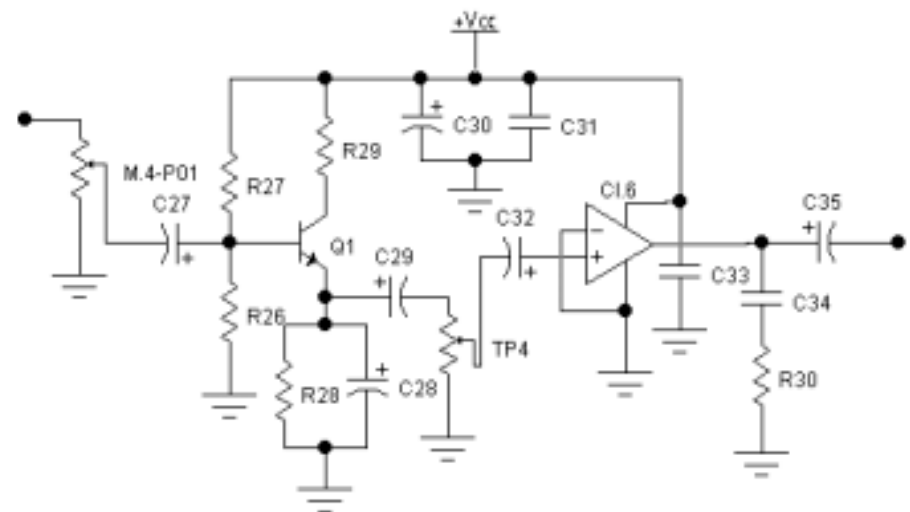
Modelo Equivalente
